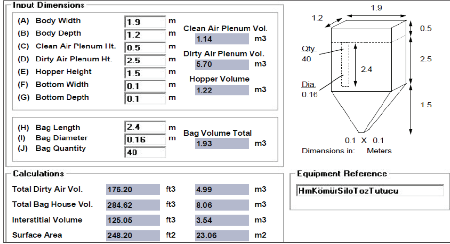
Şekil 8 – Ham Kömür Alanı Tozszulaştırmada Kullanılan Jet Filtre Ölçüleri
