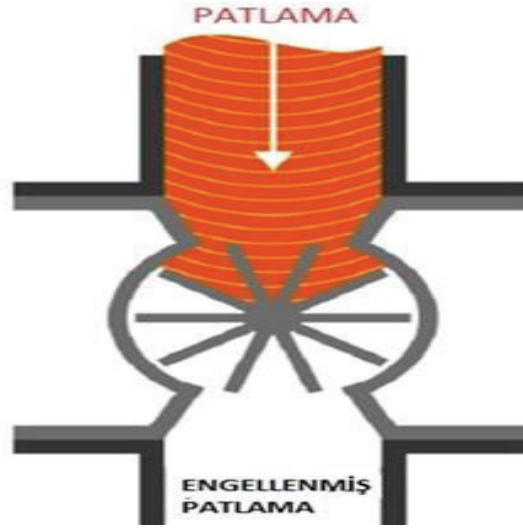
Şekil 15 – ATEX Uyumlu Hava Kilitleri
