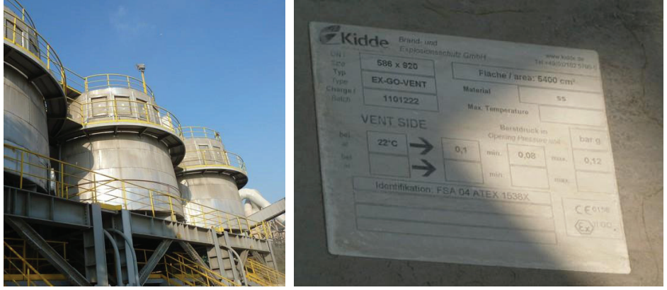
Fotoğraf 8 – ATY Silolarında Kullanılan Patlama Kapağı Örneği ve ATEX Sertifikası
