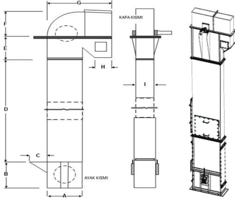
Şekil 9 – Tek Ayaklı Kovalı Elevatör
