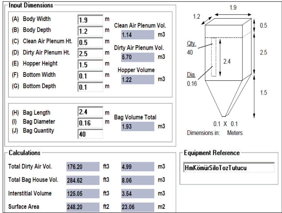
Şekil 11 – Drum seperatör jet filtresi detayları
