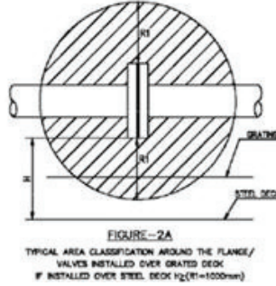
Şekil 16 – Flanj ve Vana Kaçaqları Etrafındaki Zone Sınıflandırılması Örneği
