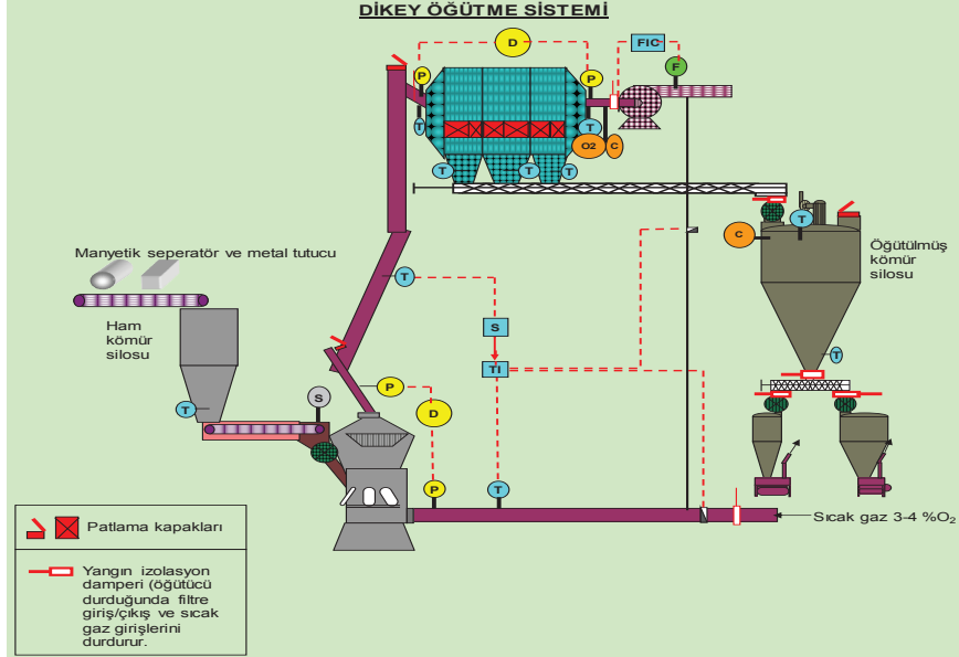
Şekil 2 – Çimento Sektöründe Tipik Kömür Öğütme Tesisi ve Ekipmanları
