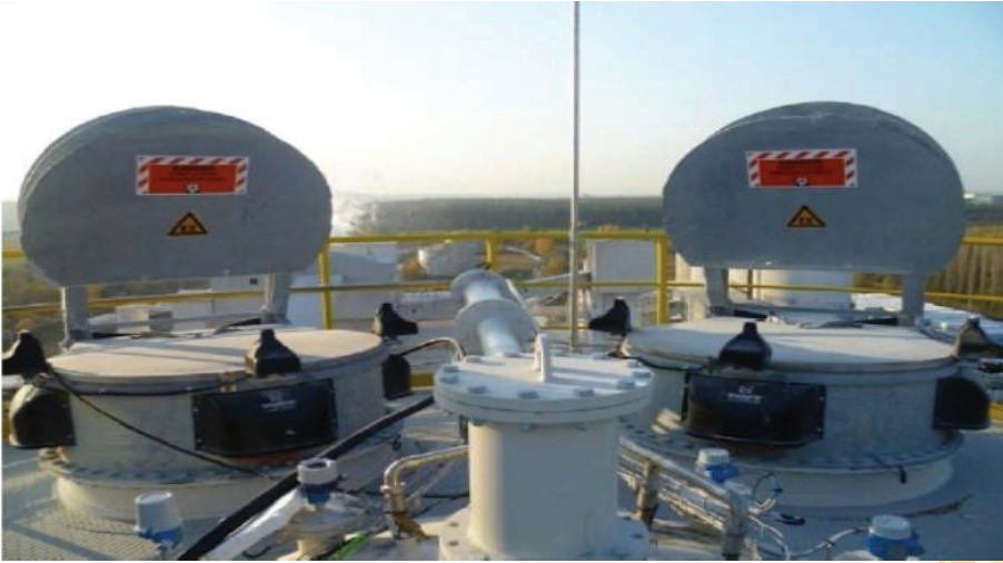
Fotoğraf 11 – Silo Üzeri Patlama Kapakları (Kendinden Kapanan ve Vakum Kırıcılı) 23
